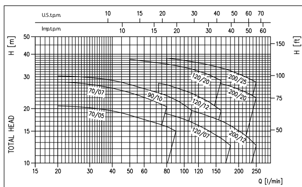
GAMME DE PERFORMANCES (selon ISO 9906 Annexe A)
