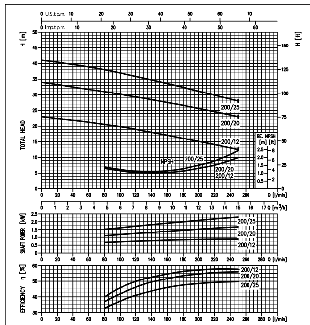
COURBES DE PERFORMANCE série PCX200 (selon ISO 9906 Annexe A)
