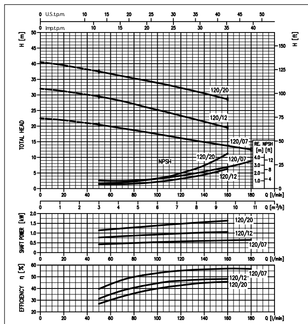
COURBES DE PERFORMANCE série PCX120 (selon ISO 9906 Annexe A)
