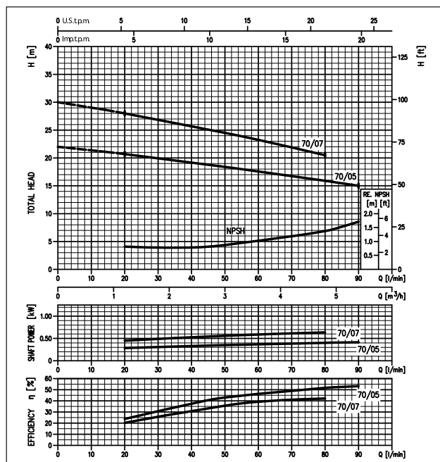
COURBES DE PERFORMANCE série PCX70 (selon ISO 9906 Annexe A)
