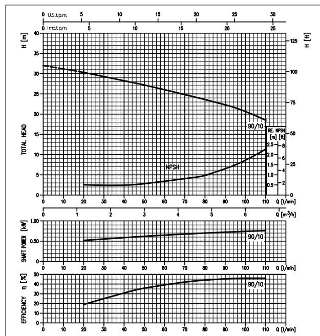
COURBES DE PERFORMANCE série PCX90 (selon ISO 9906 Annexe A)
